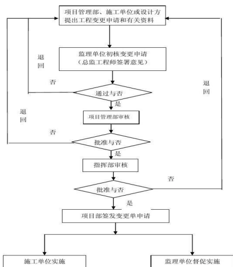
图2 工程变更流程图
