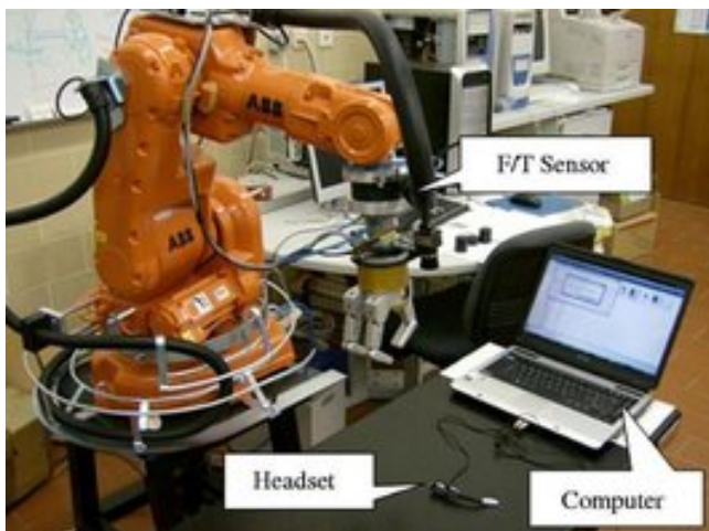
图1 工业机器
