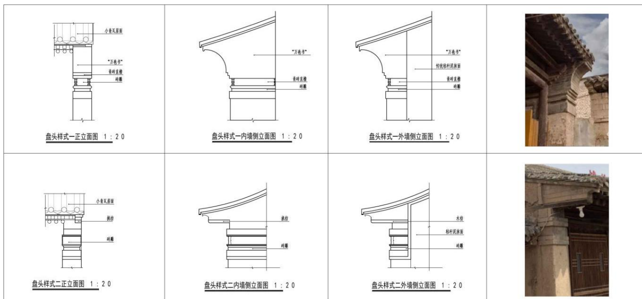
图2 传统民居建筑盘头对比图
