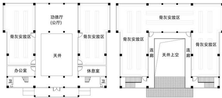
图3 骨灰楼一层、二层平面图
