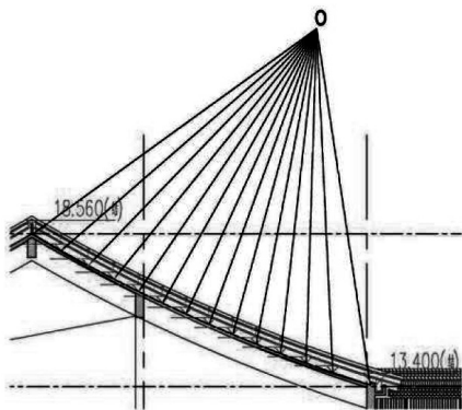
图 4-2 弧形屋面以直代曲分割图
