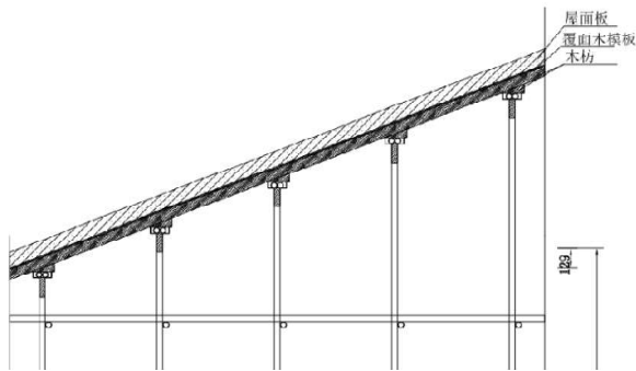
图 4-1 模板支撑架大样图
