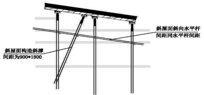
图 4-5 斜屋面增设斜撑及斜向水平杆做法
