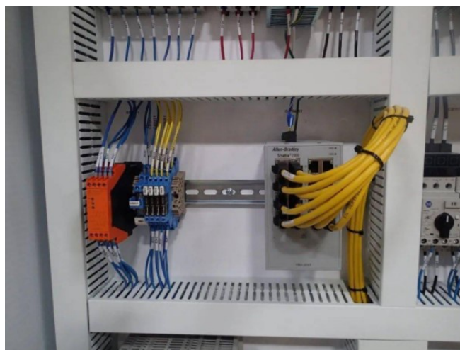
图1 配电柜内布线
