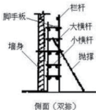
图2 脚手架布置形式
