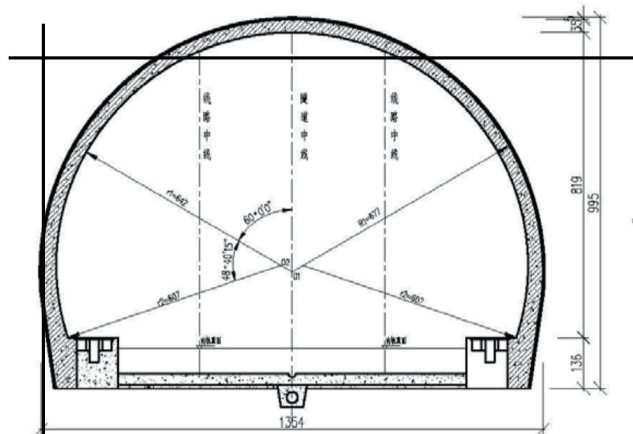
图3 广深港客运专线隧道横断面图
