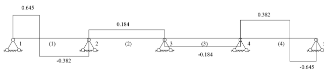
图7 主梁剪力图 (kN)
