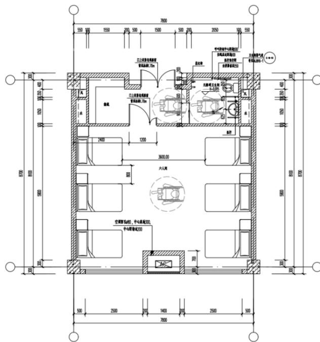
六人间 放大平面图 1:50
