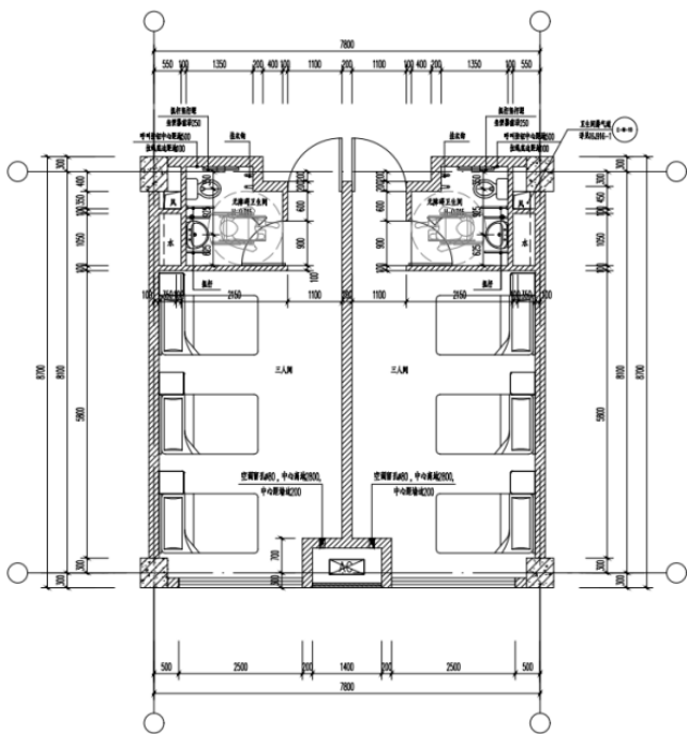
三人间 放大平面图 1:50
