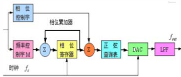
图1 波形信号发生器
