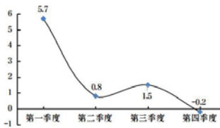
图2 2022年我国居民人均消费支出累计增长率
