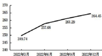
图1 2022年我国本外币存款余额（单位：万亿元）
