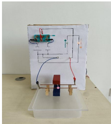
图1 安培力方向探究仪
