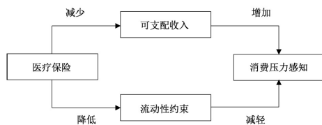
图2 医疗保险影响消费压力感知的机制分析
