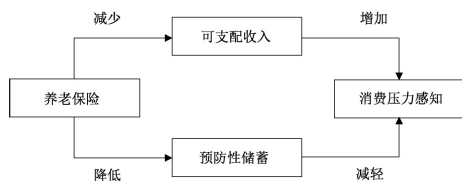
图1 养老保险影响消费压力感知的机制分析
